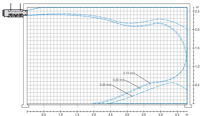
Diagramm 11. Seitenansicht A-A – Luftgeschwindigkeit für Lamellenstellung, 0°.
