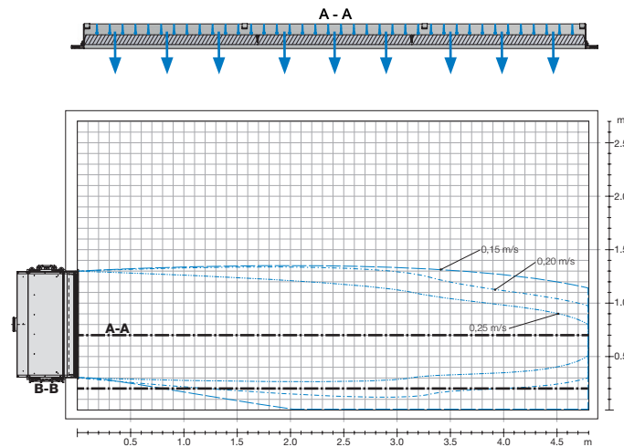
Diagramm 10. Ansicht von oben – Luftgeschwindigkeit für Lamellenstellung 0°.
