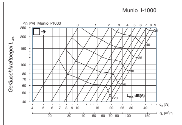
Diagramm 6.b. Schalleistungspegel L_{WA} Munio I-1000.
