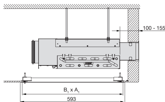
Abbildung 25. Montagezeichnung für Frontplatte -3S mit Ausschnittmaßen.
