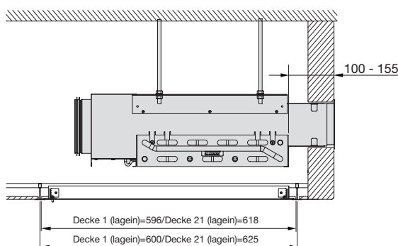
Abbildung 26. Montagezeichnung für Frontplatte -01/-21 mit äußeren Maßen.
