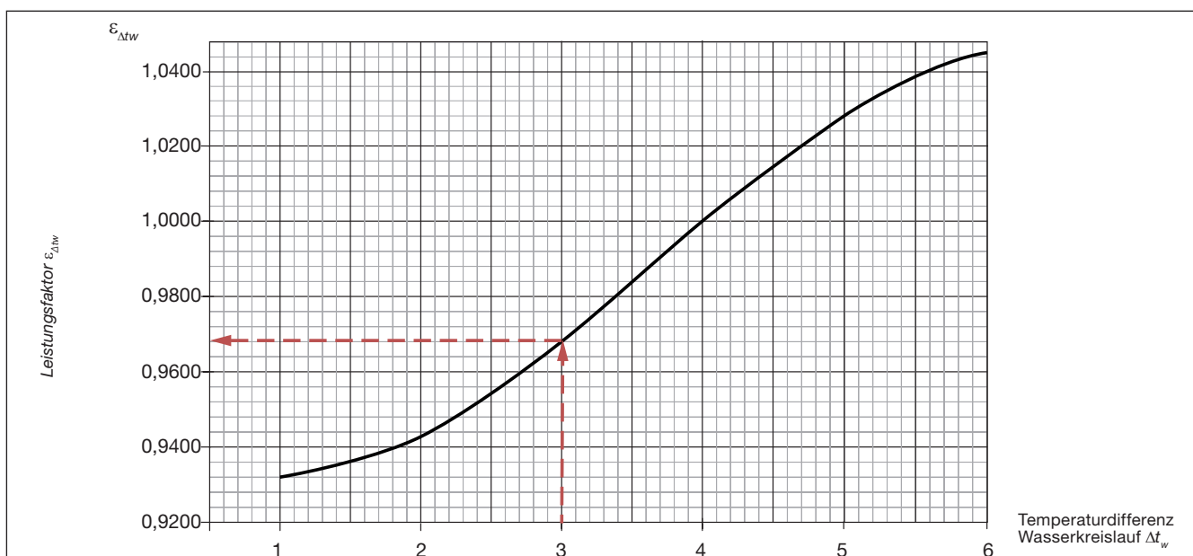
Diagramm 3. Leistungsfaktor \varepsilon_{\Delta t_w} als Funktion von \Delta t_w . Gilt nur für Kühlen.
