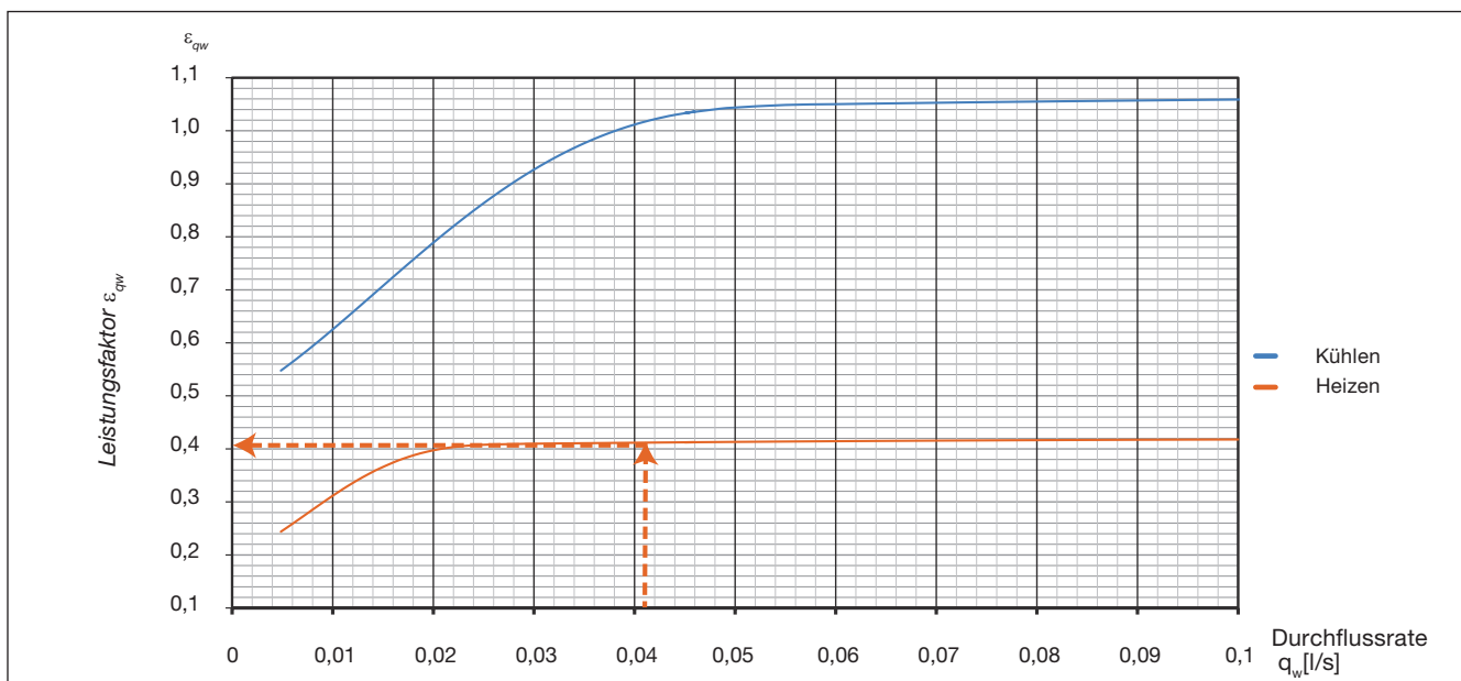
Diagramm 4. Leistungsfaktor \varepsilon_{qw} für Wasserdurchfluss (Heizen und Kühlen).
