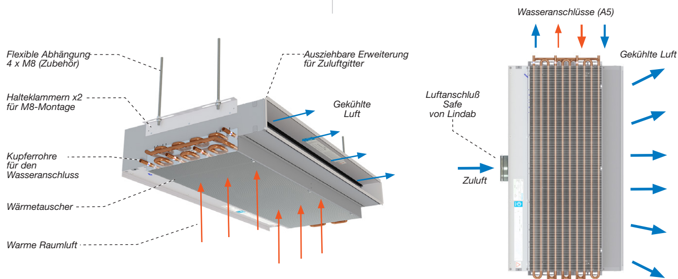
Abbildung 2a/b. Teile und Funktionsprinzip des Standard Munio-I-1000 (ohne Frontplatte).
