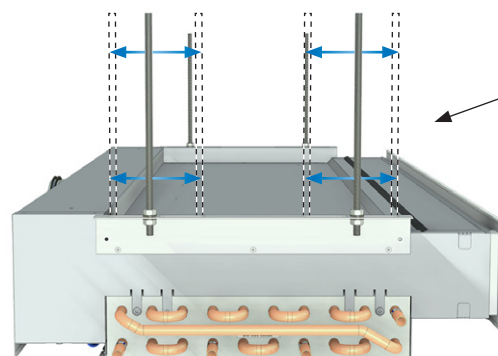
Abbildung 19. Munio-I Abhängung, Verschiedene Abhängertypen sind als Zubehör verfügbar.
