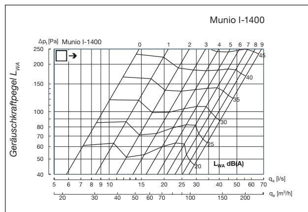
Diagramm 6.d. Schalleistungspegel L_{WA} Munio I-1400.
