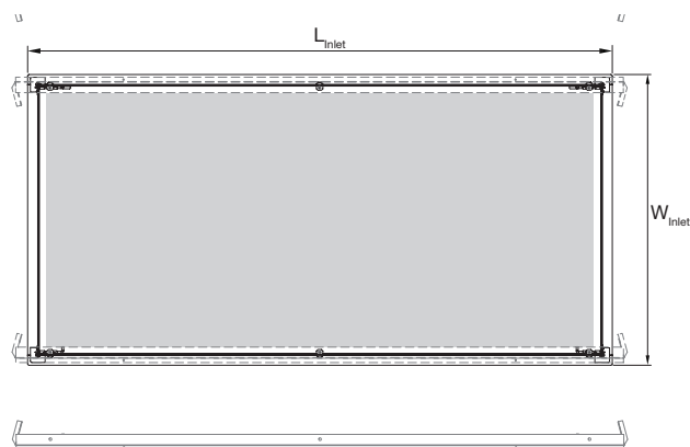
Abbildung 22. Frontplatte -3S Maße.
