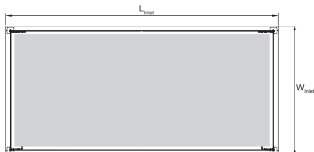
Abbildung 23. Frontplatte -01/-21 Maße.
