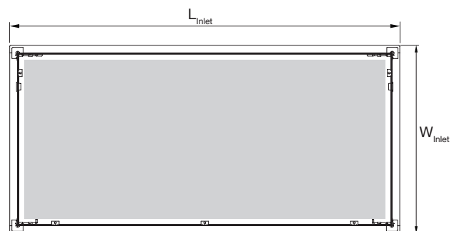
Abbildung 21. Maße Frontplatte -03 (für -3E siehe „Montageanleitung“).
