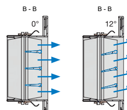
Abbildung 8a. Horizontale Lamellen in neutraler Position ( 0^\circ ) und Umlenkung von 12^\circ .
