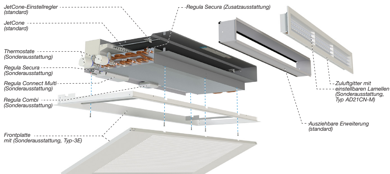
Abbildung 3. Munio-I mit einigen Sonderausstattungen.
