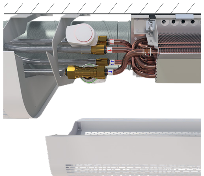
Abbildung 8. Plafond XD mit Abdeckung Clyp in Reihe.
