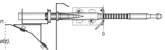
Abbildung 19. Positionen und Einstellungen der Einstellstifte.
