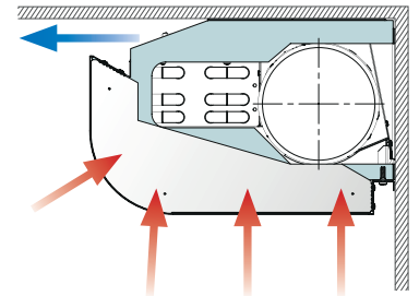
Abbildung 11. Plafond XD-FC Montage an der Wand, bündig zur Decke (FC).
