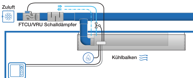
Abbildung 47. Plafond XD mit FTCU und Schalldämpfer.
