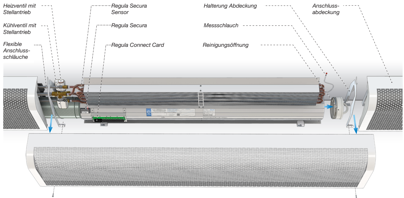
Abbildung 81. Plafond XD mit Designabdeckung Typ Ctyp. Die Abdeckung lässt sich zu Wartungszwecken leicht abnehmen, während die Anschlussabdeckungen an Ort und Stelle bleiben. Hier wird die Perforation der Anschlussabdeckungen durch schwarzes Vlies auf der Innenseite der Abdeckungen verschlossen (nicht im Lieferumfang enthalten).
