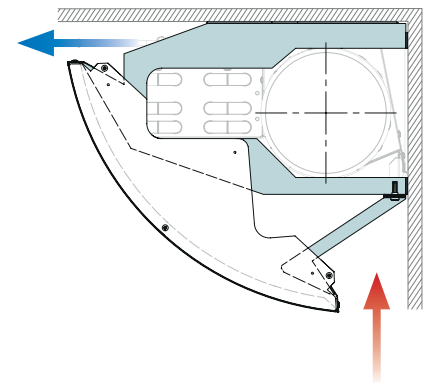
Abbildung 35. Plafond XD, die Badge Abdeckung ist das einzige Design, das keine Perforation, sondern einen offenen, sichtbaren Schlitz für den Raumlufteinlass hat.
