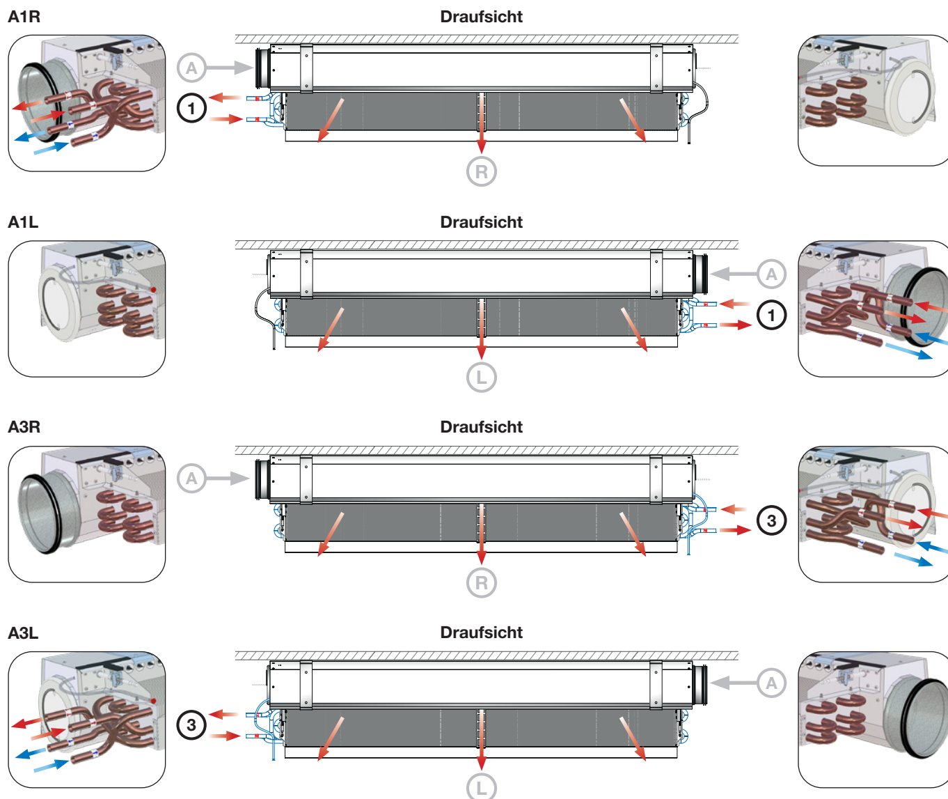
Abbildung 78. Identifizierung der Wasseranschlüsse für den 4-Wege-Wasserkreislauf des Plafond XD Gehäuses.
