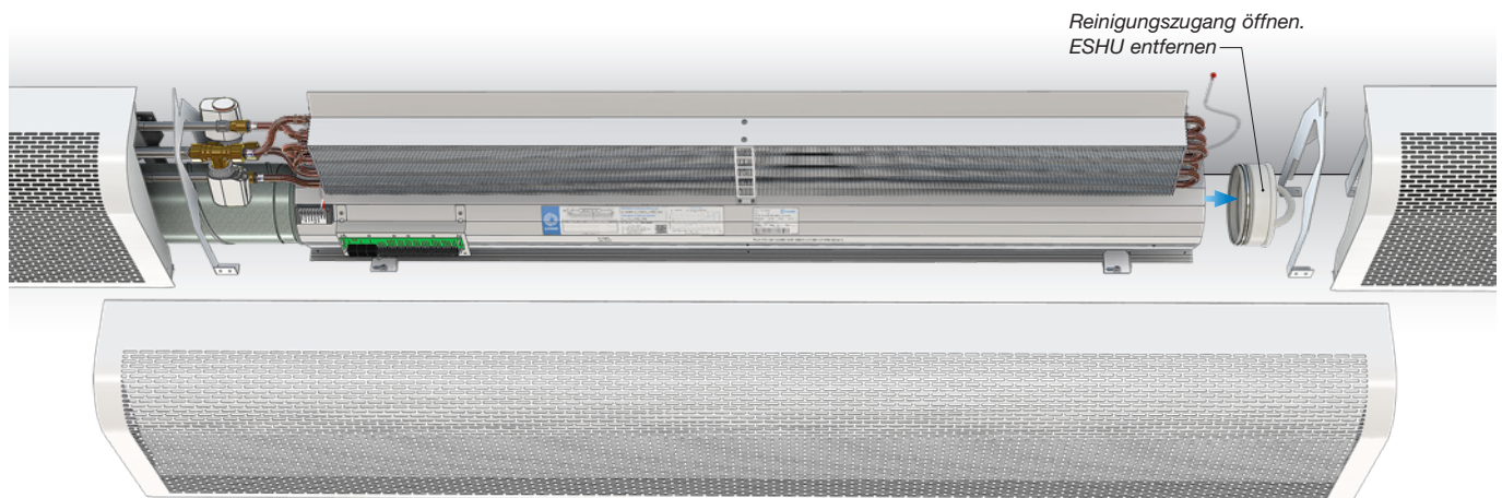
Abbildung 44. Leichter Zugang zum Balkengehäuse. Alles ist zugänglich.
