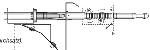
Pos. 0 Max. geschlossen. Einstellung der Düse (20% Luftdurchsatz).
