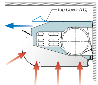
Abbildung 13. Plafond XD-FW Montage an der Wand, mit Abstand zur Decke (FW).
